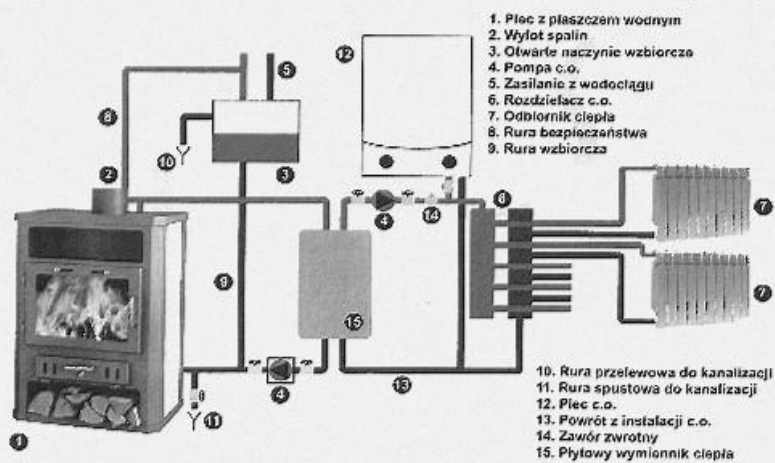
Schemat podłączenia pieca z płaszczem wodnym z kotłem gazowym
